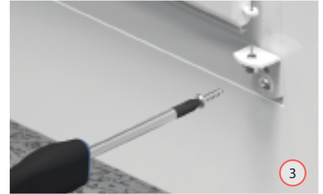
OPTIONEEL - schroef de spanhoek tegen de wand of het kozijn
